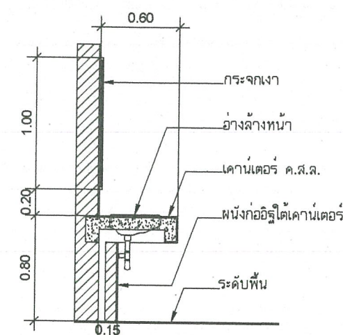
อ่างล้างหน้าชนิดฝังเคาน์เตอร์
