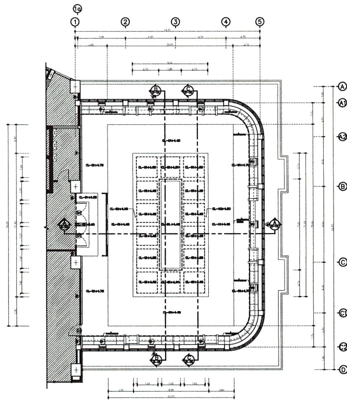
แปลนฝ้าเพดาน Scale 1:100
