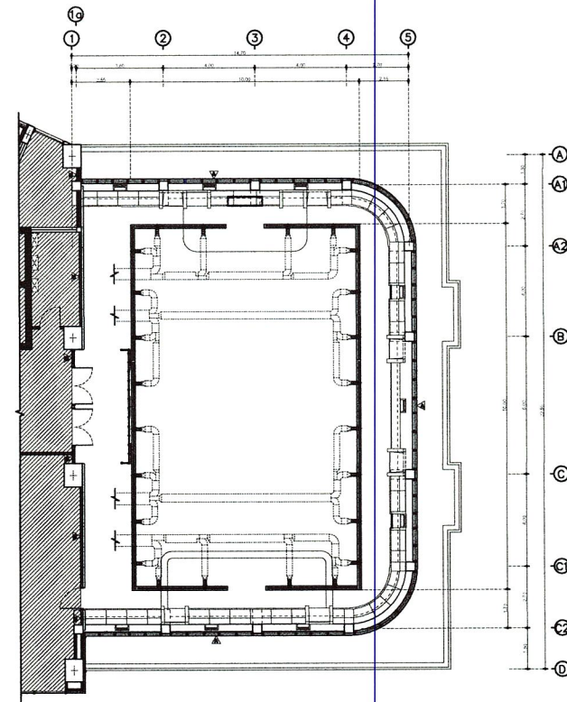
ผังแสดงตำแหน่งเครื่องปรับอากาศ Scale 1:100
