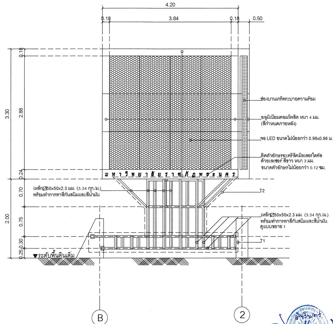
รูปด้าน 1 ป้าย LED Screen System มาตราส่วน 1:50
