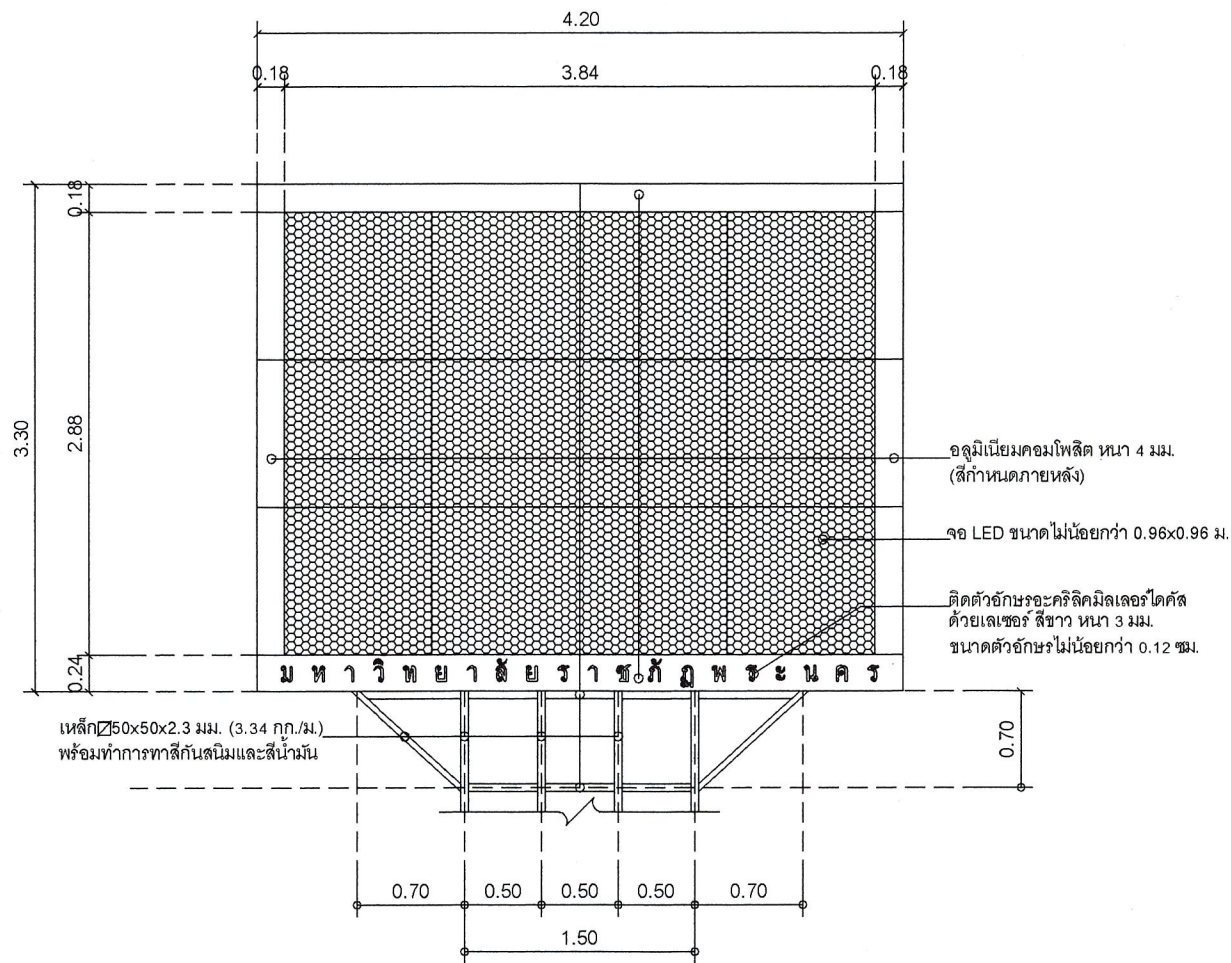
รูปด้านหน้าป้าย LED Screen System มาตราส่วน 1:50
