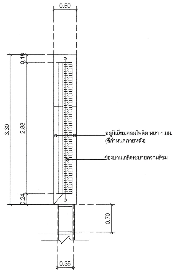
รูปด้านข้างป้าย LED Screen System มาตราส่วน 1:50
