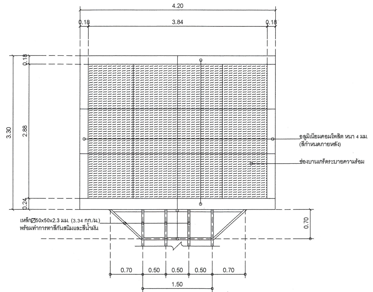
รูปด้านหลังป้าย LED Screen System มาตราส่วน 1:50
