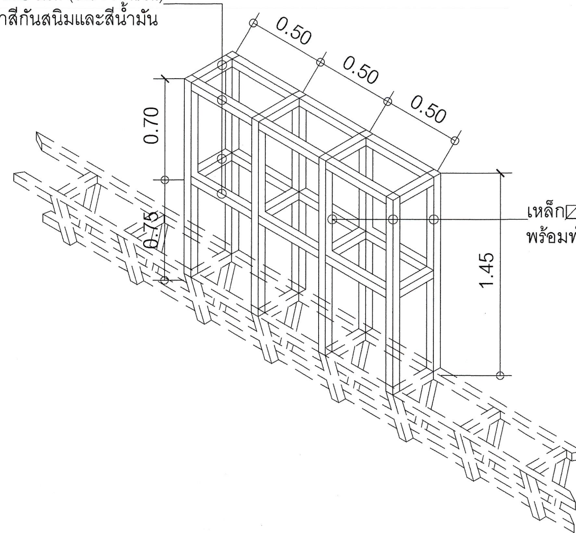
แบบขยาย 1 (T2) มาตราส่วน 1:50
