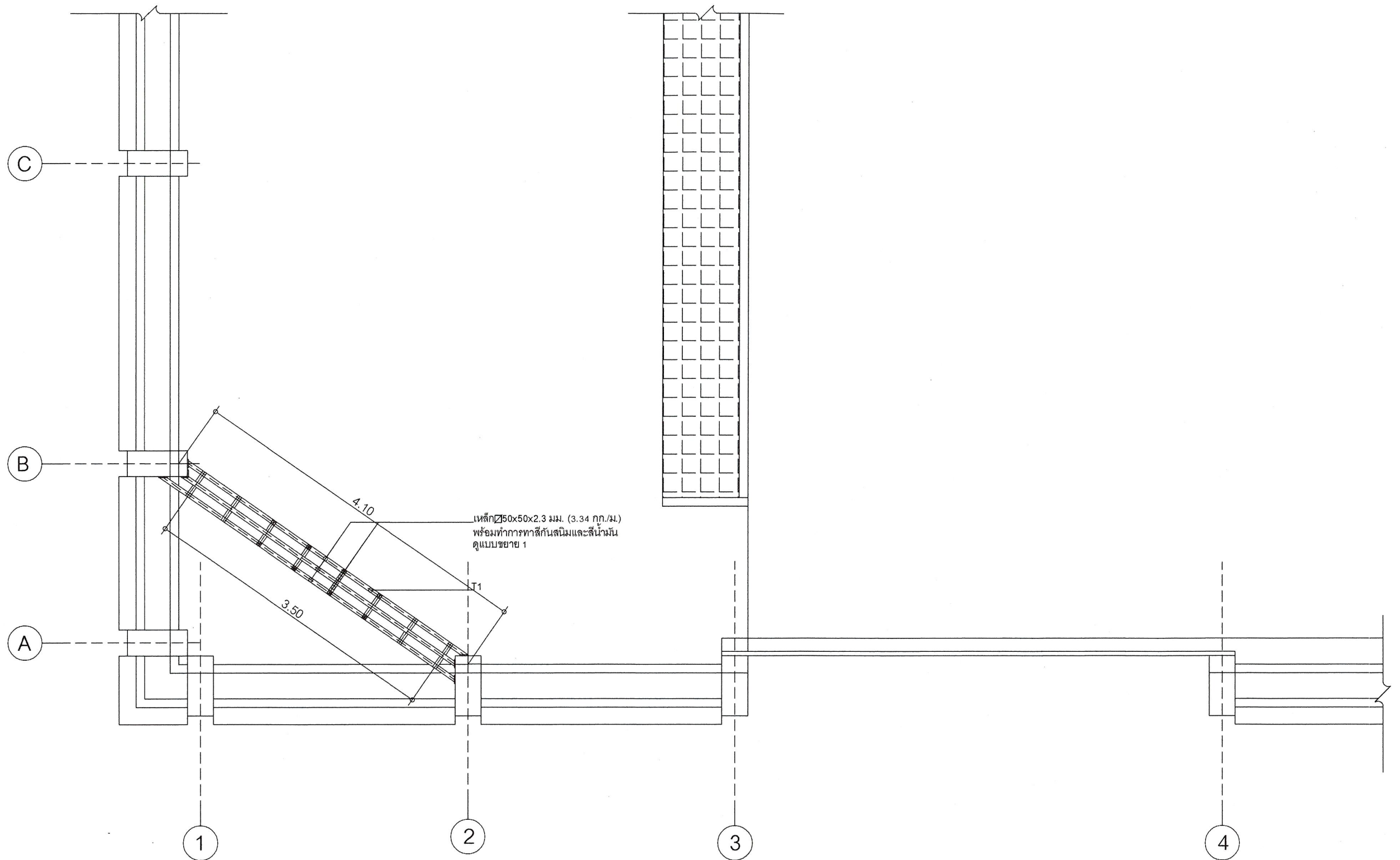
แบบแปลนโครงสร้างป้าย LED Screen System มาตราส่วน 1:50
