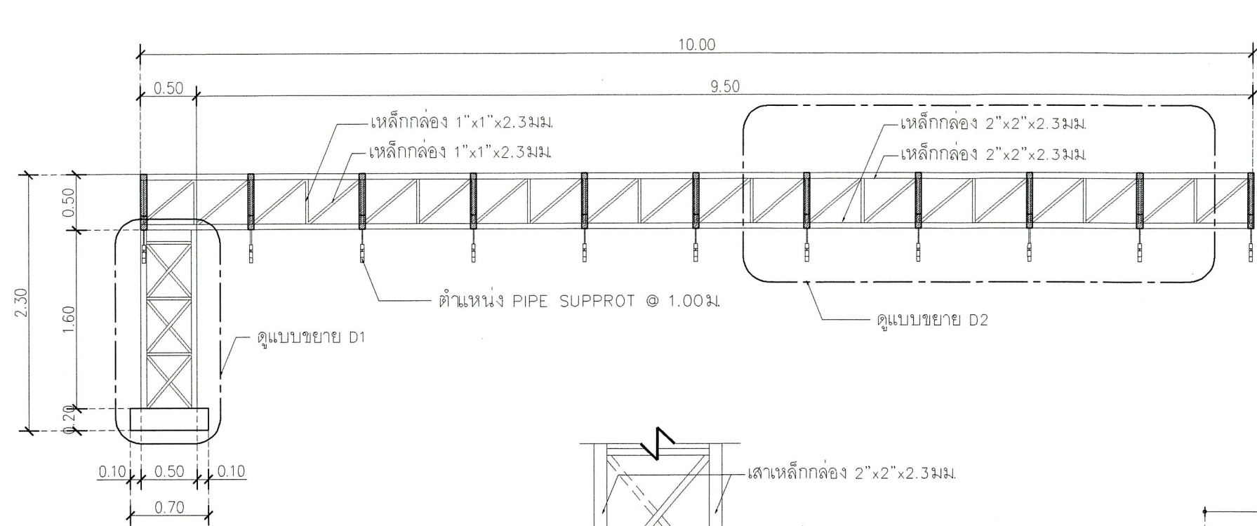
แปลนแบบขยาย โครงเหล็ก ชั้นหลังคา ห้อง PUMP ROOM มาตราส่วน 1:50
