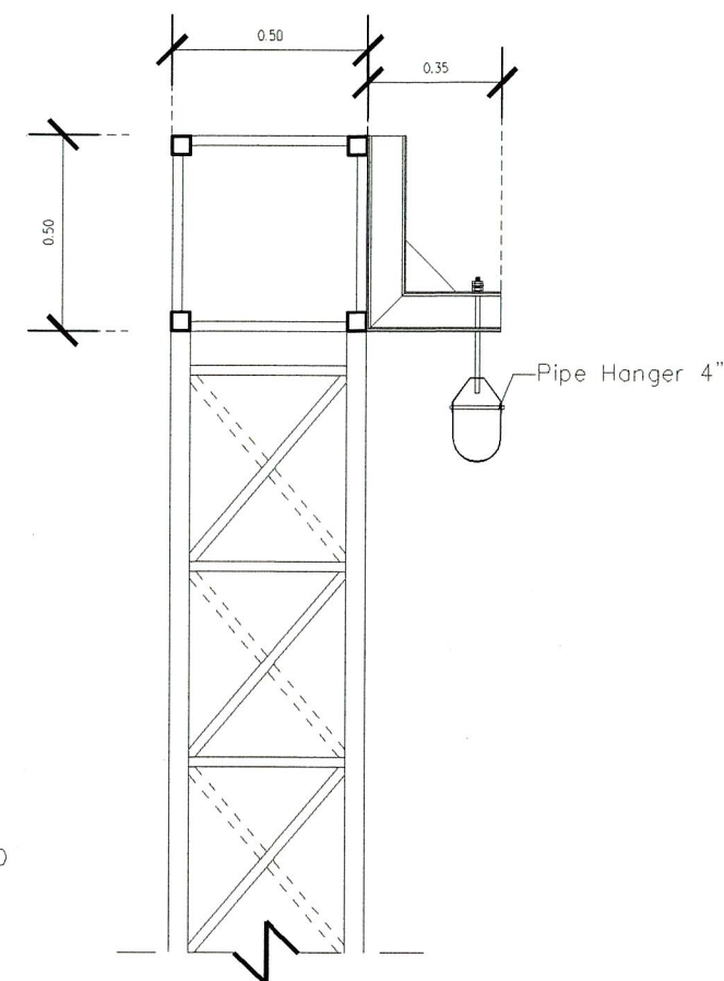
แบบขยาย PIPE SUPPROT มาตราส่วน NONE
