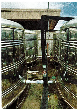
CWด1"แนวตั้งจากหลังประตุน้ำ(ของเดิม)เข้าถังน้ำดีเปลี่ยนใหม่ ชนิด PPR พร้อมฉนวนหุ้ม
