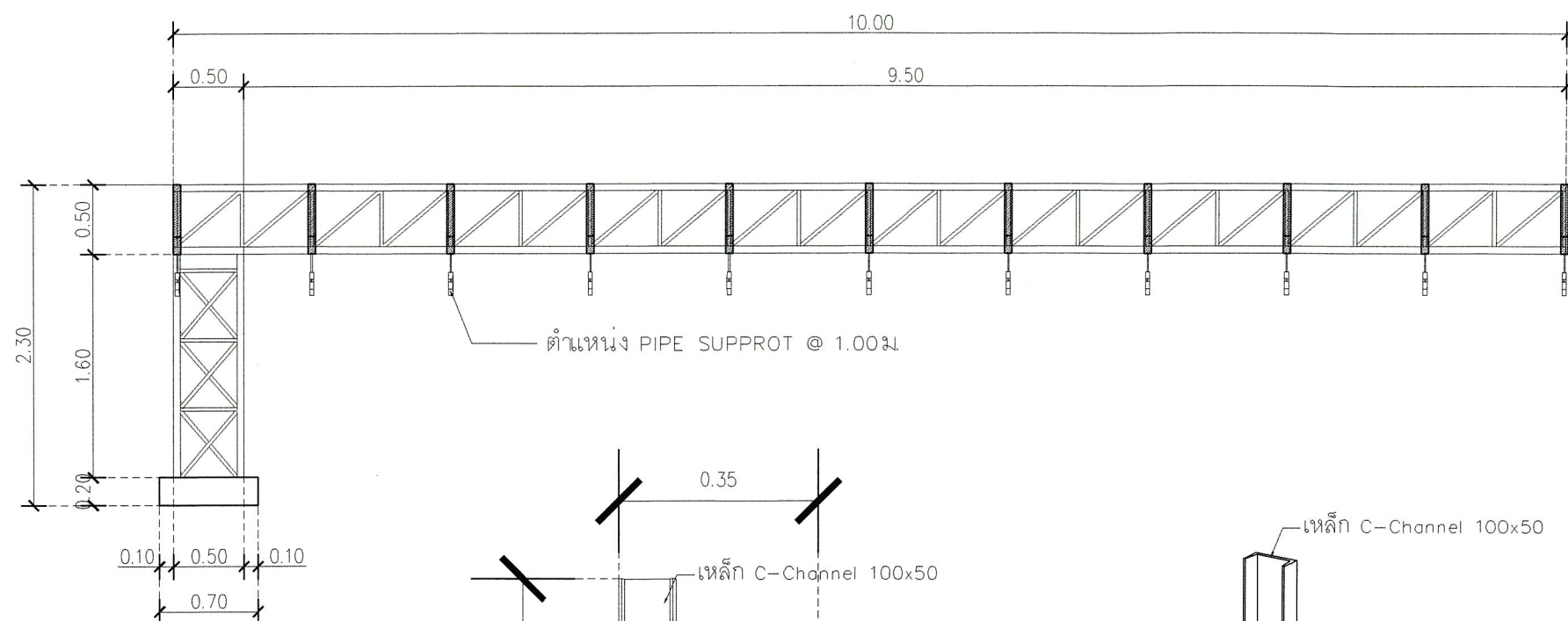
แปลนแบบขยายตำแหน่ง PIPE SUPPROT มาตราส่วน 1:50
