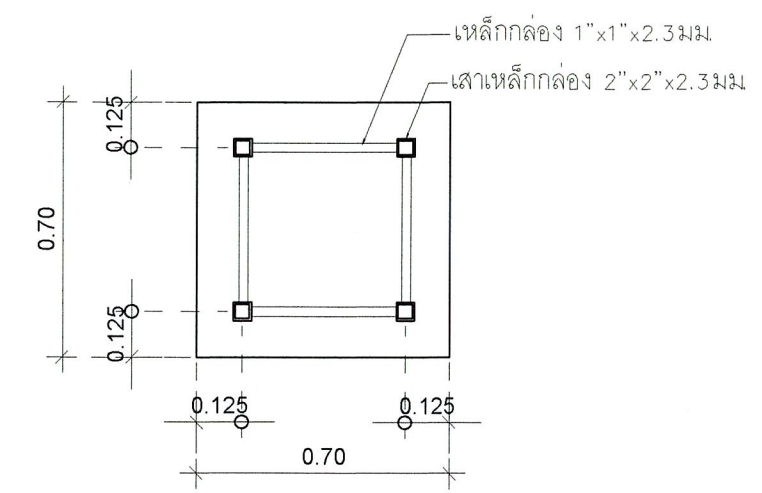
แปลนแบบขยาย ฐานโครงเหล็ก มาตราส่วน 1:25
