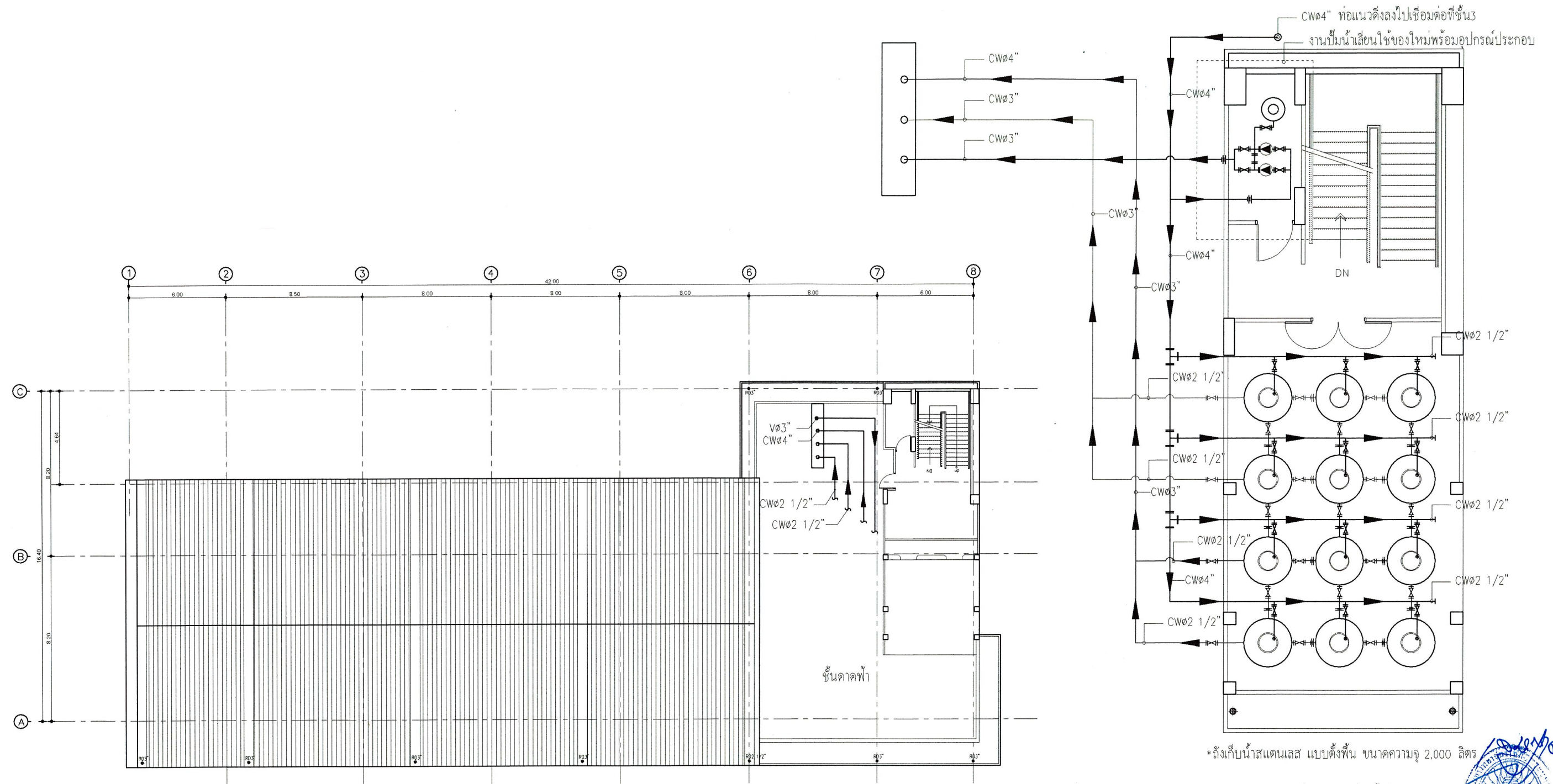
SANITARI AND FIRE PROTECTION SYSTEM ROOF PLAN มาตราส่วน 1 : 250
