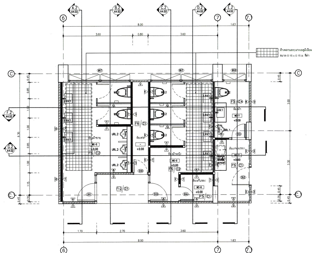
แปลนแบบขยาย ห้องน้ำชั้นที่ 5,6,7,9,10
