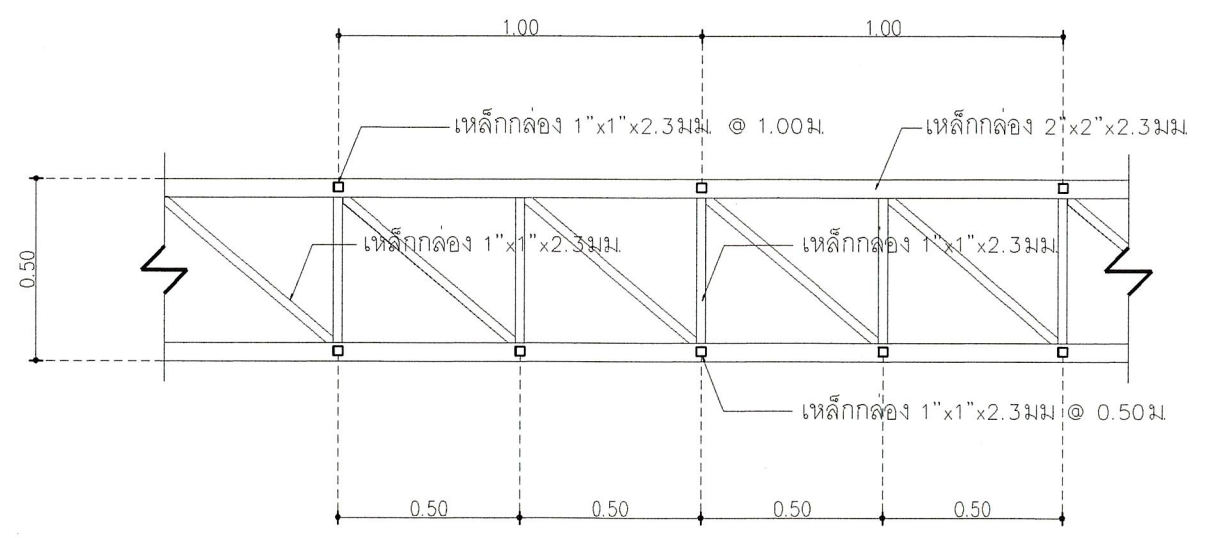
แปลนแบบขยาย โครงเหล็ก D2 มาตราส่วน 1:25
