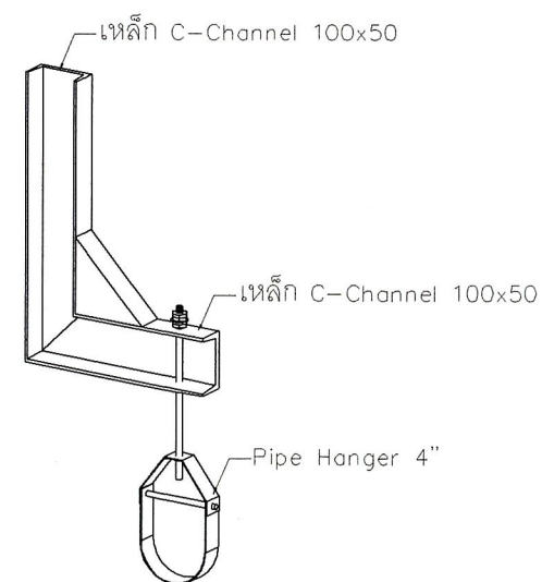
แบบขยาย PIPE SUPPROT มาตราส่วน NONE
