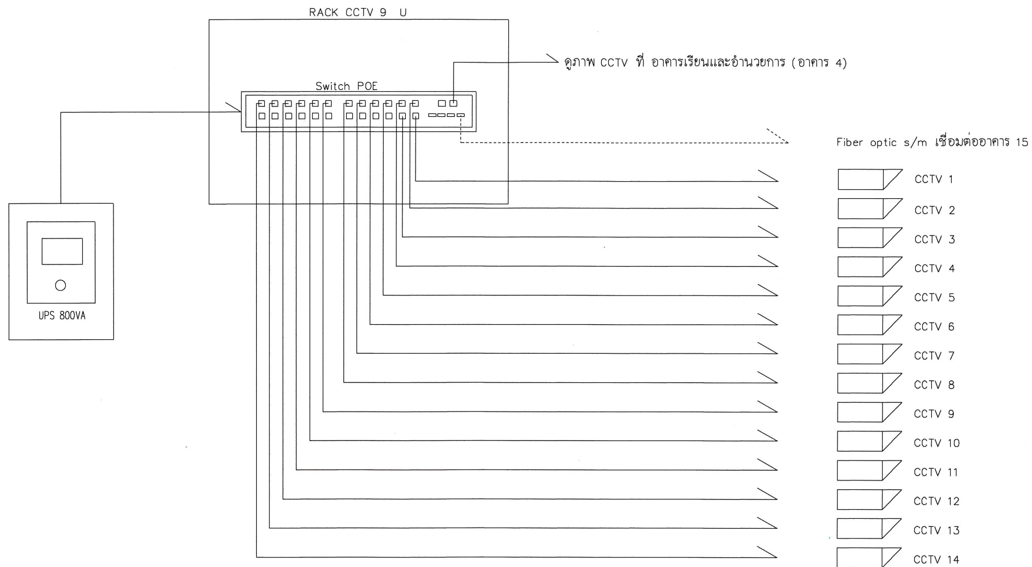
Diagram ระบบกล้องวงจรปิด CCTV IP NETWORK มาตราส่วน /SCALE 1:100
