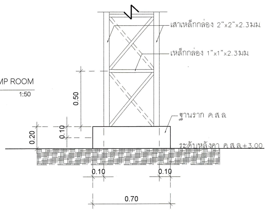
แปลนแบบขยาย โครงเหล็ก D1 มาตราส่วน 1:25
