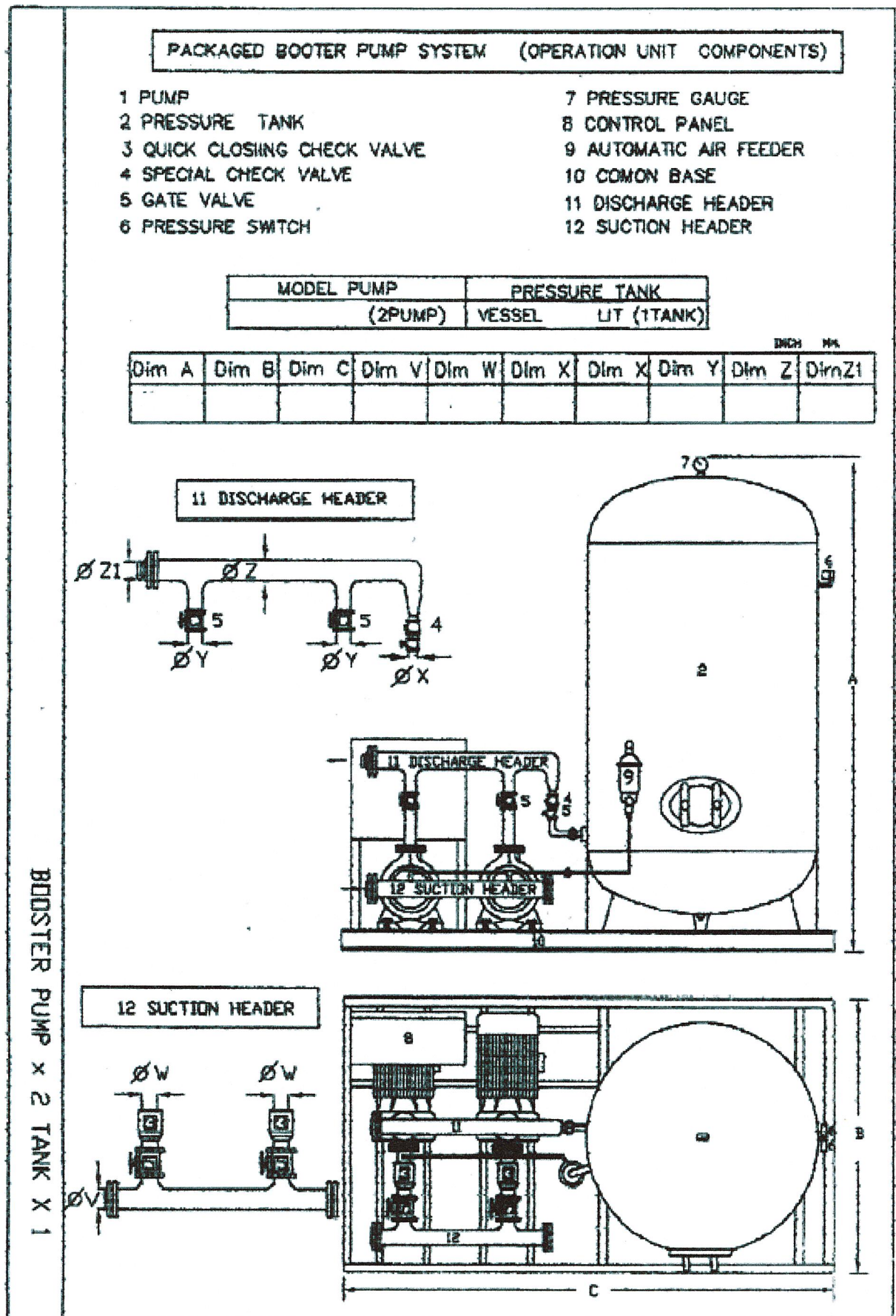
ภาพที่ 1 ตัวอย่าง Package Booster Pump System
