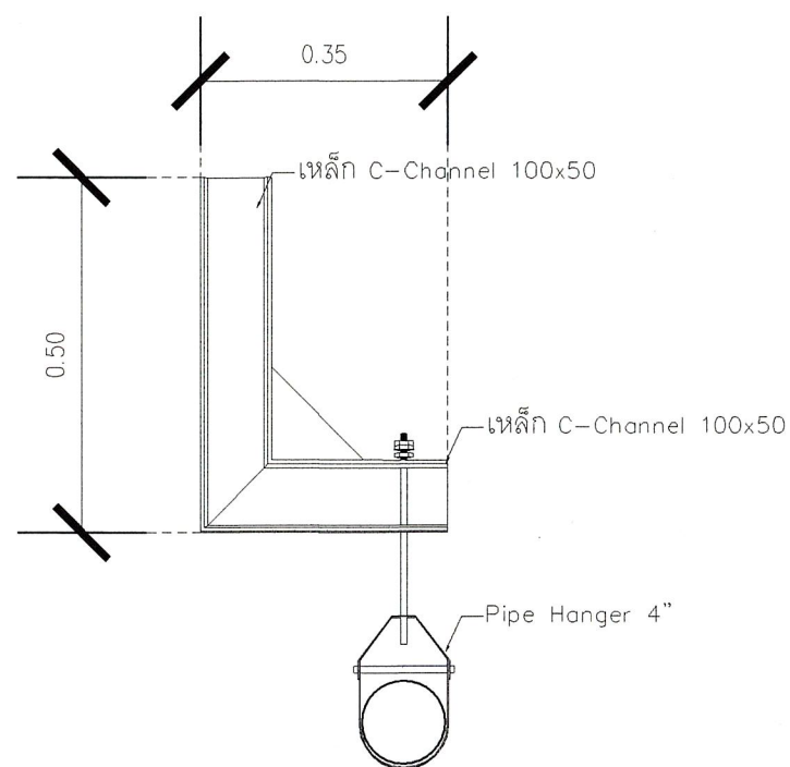
แปลนแบบขยายตำแหน่ง PIPE SUPPROT มาตราส่วน 1:50
