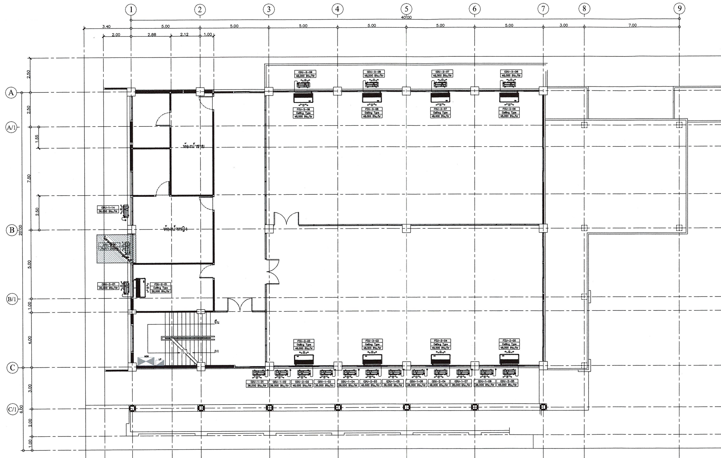
แบบแปลนพื้นชั้น 2 มาตราส่วน 1:150
