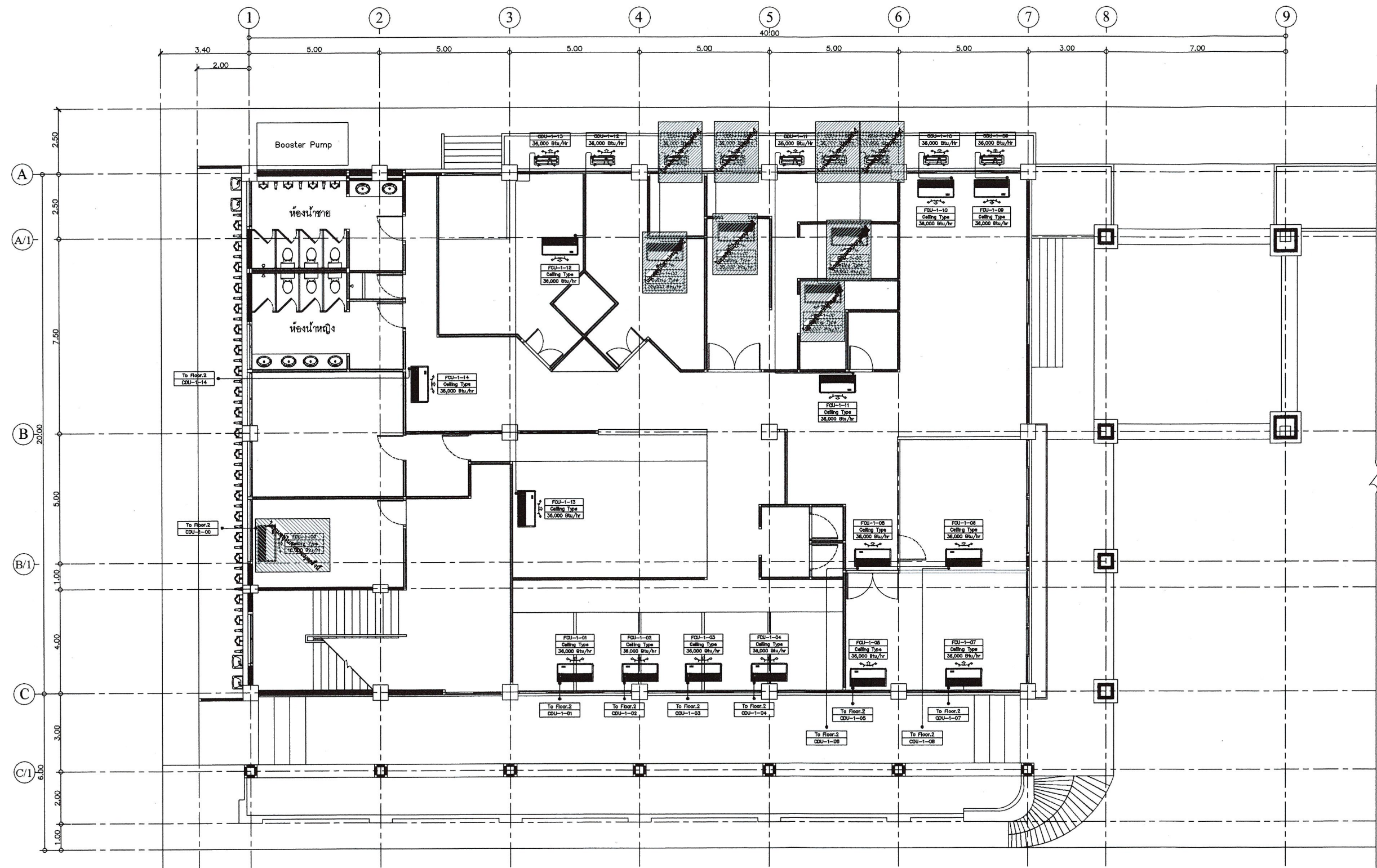
แบบแปลนพื้นชั้น 1 มาตราส่วน 1:150
